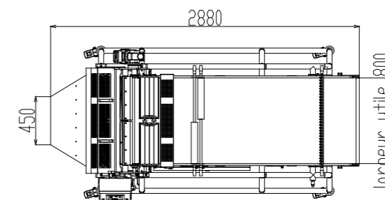
Plans du modèle CUX-800
